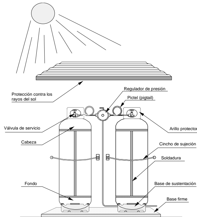
Figura 1. - Instalación típica para cilindros portátiles
